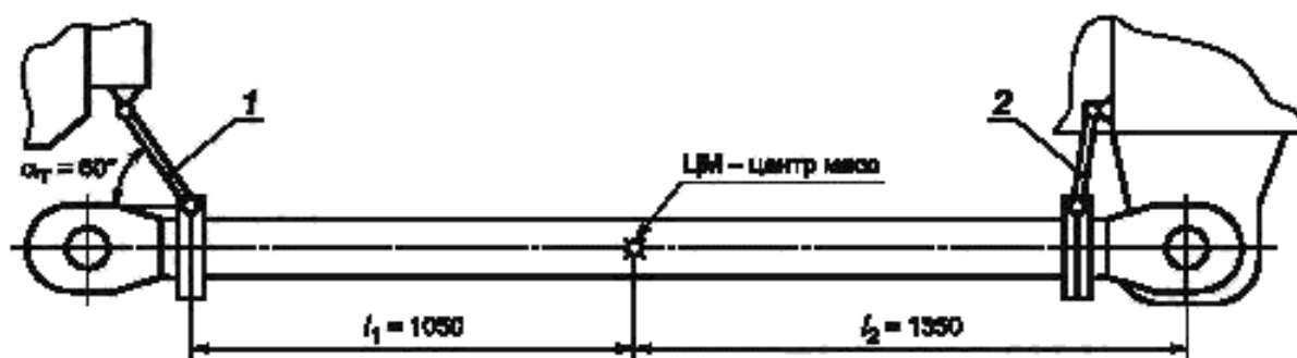
1 — страховочный канат опоры 1; 2 — страховочный канат опоры 2
