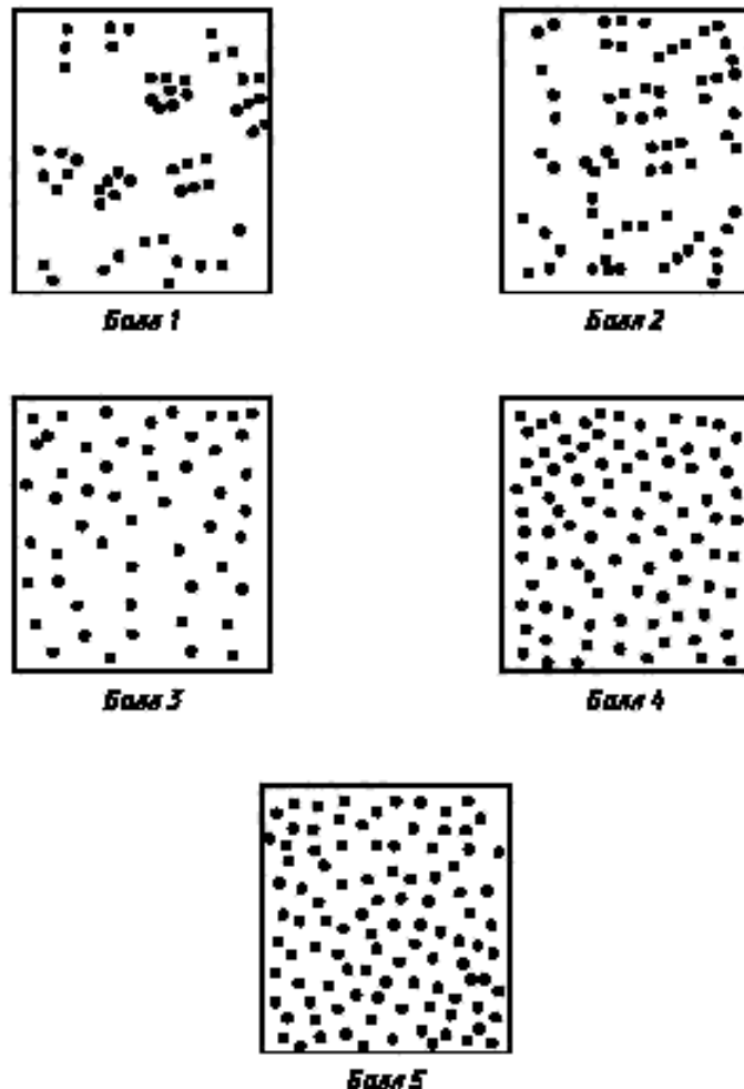
Рисунок Б.1 — Шкала пористости алюминиевых сплавов
