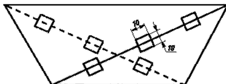
Рисунок Б.2 — Схема расположения квадратов на макрошлифе
