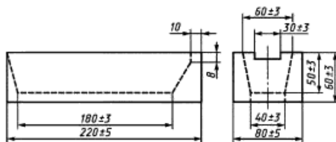
Рисунок 1 — Изложница
