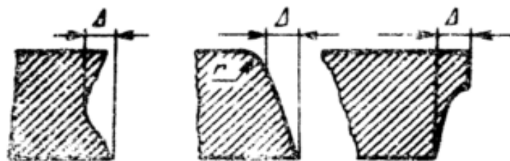
\Delta — отклонение поверхности реза от перпендикулярности
