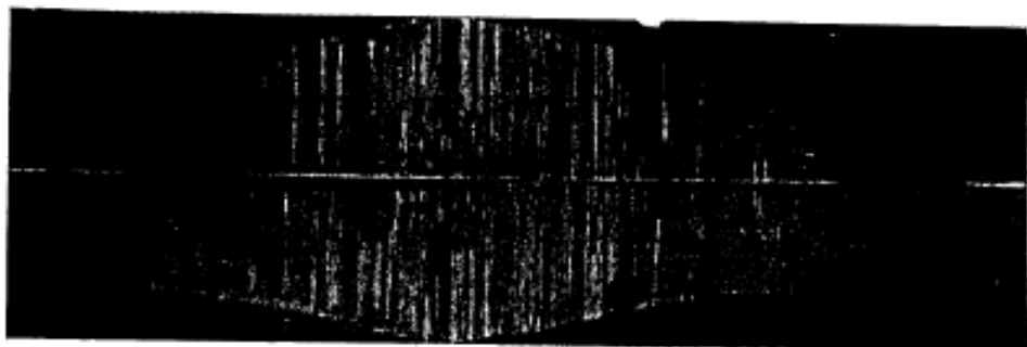
a — слоистый излом в осевой части заготовки
